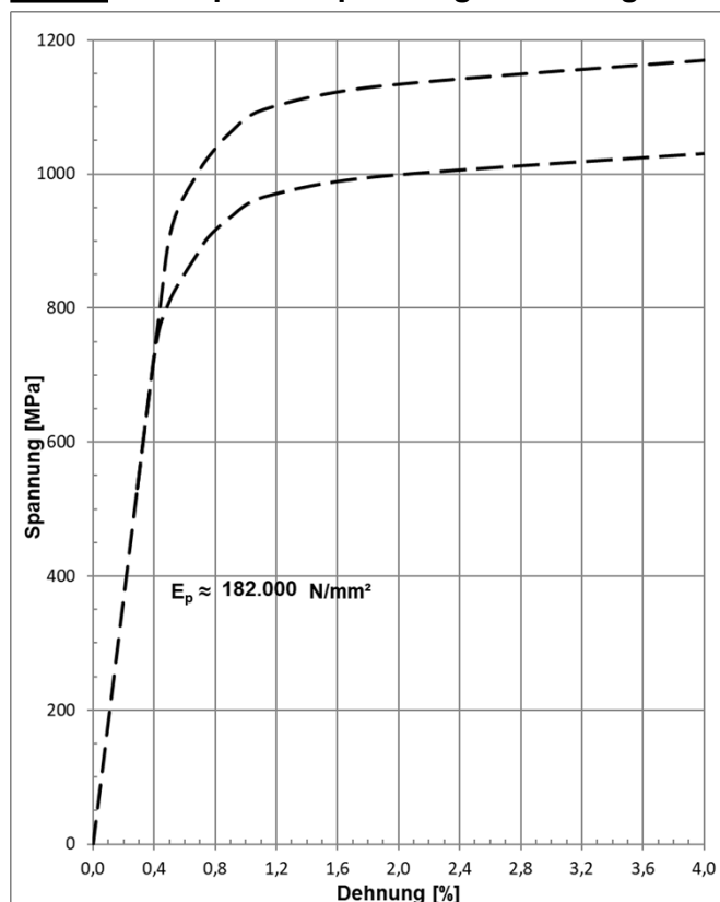
Bild 2: Prinzipieller Spannungs-Dehnungsverlauf
